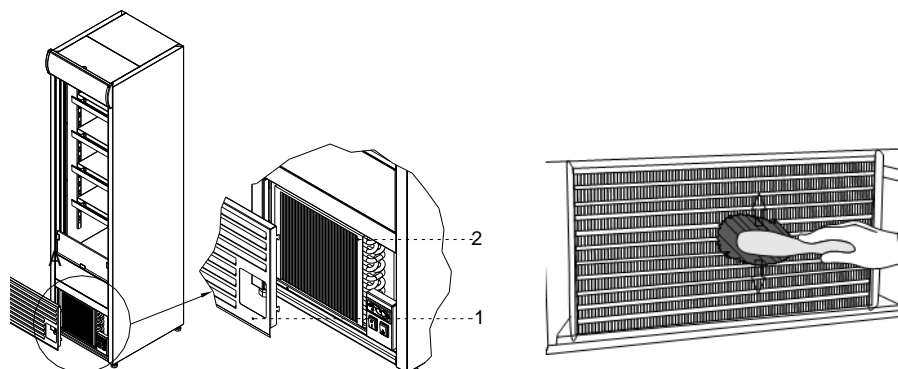
Rys.5 Czyszczenie skraplacza
