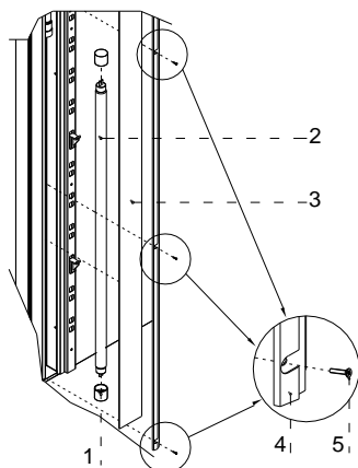
Rys.6 Wymiana świetlówki wewnątrz szafy
