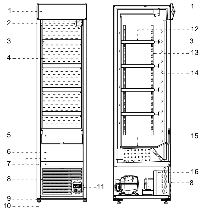
Rys.1 Budowa urządzenia
