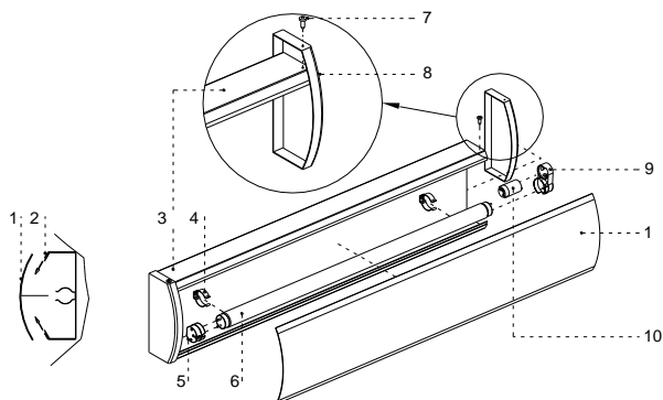
Rys.7 Wymiana świetlówki panelu górnego
