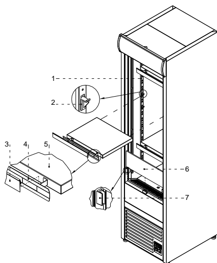
Rys.3 Mocowanie półki ekspozycyjnej i ekranu frontowego
