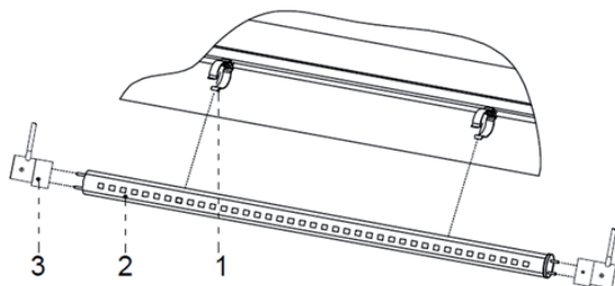
Rys. 5. Wymiana świetlówki LED
