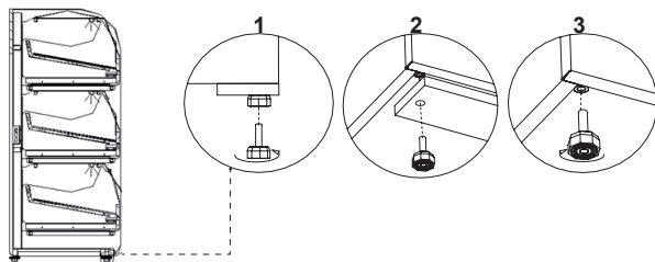
Rys. 2. Usuwanie podestu drewnianego
