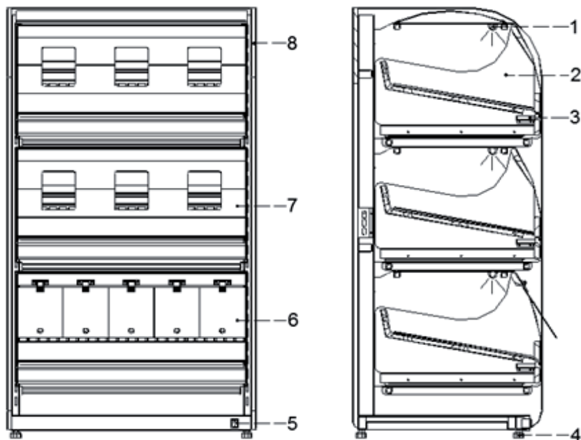
Rys. 1. Budowa urządzenia
